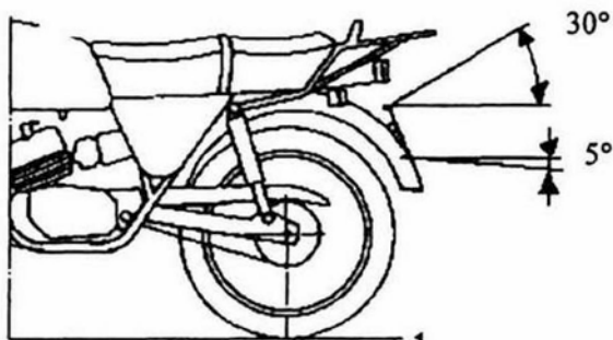
ANGOLO DI VISIBILITA' GEOMETRICA (DIEDRO CON SPIGOLO ORIZZONTALE) ANGLE OF GEOMETRIC VISIBILITY (DIEDRAL WITH HORIZONTAL EDGE)
